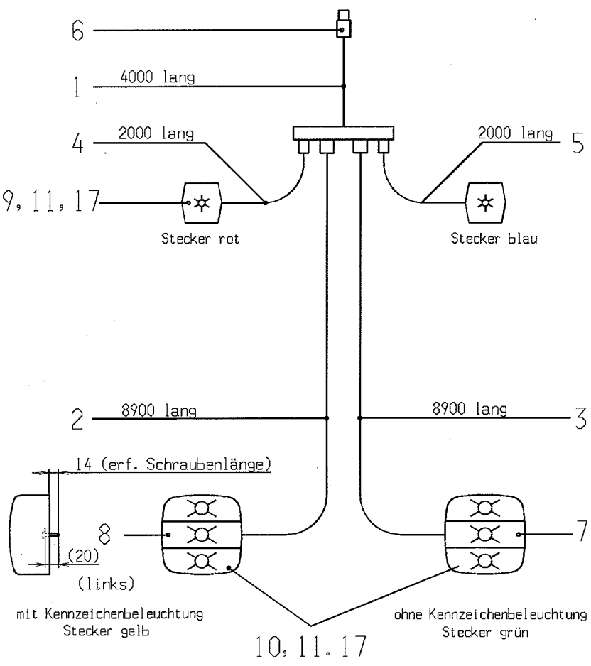
Nennspannung 12 V schematische Darstellung
